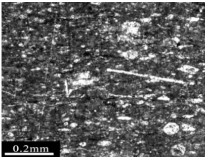
含泥含棘皮动物碎屑粒泥灰岩
