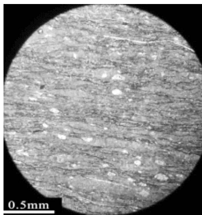
深色层状含有机质泥粒灰岩
