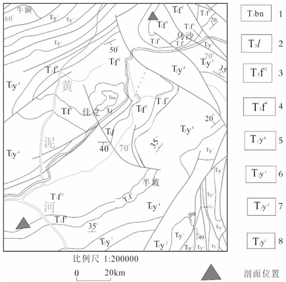
图1 兴义乌沙地质简图(清绘自1:200000罗平幅)
