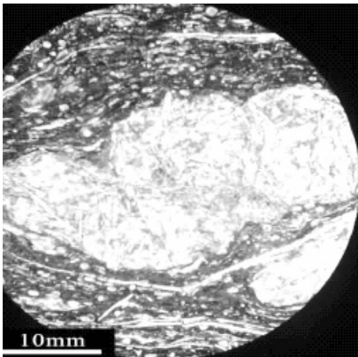
含藻屑含薄壳远洋双壳类粒泥灰岩
