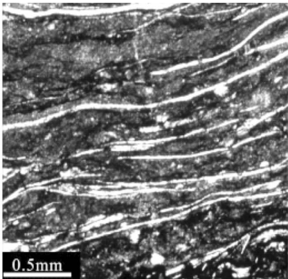
含藻屑含薄壳远洋双壳类粒泥灰岩
