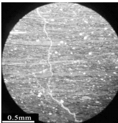
深色层状含有机质泥粒灰岩
