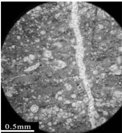
含完整生物化石的粒泥灰岩
