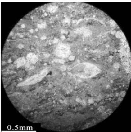
含完整生物化石的粒泥灰岩
